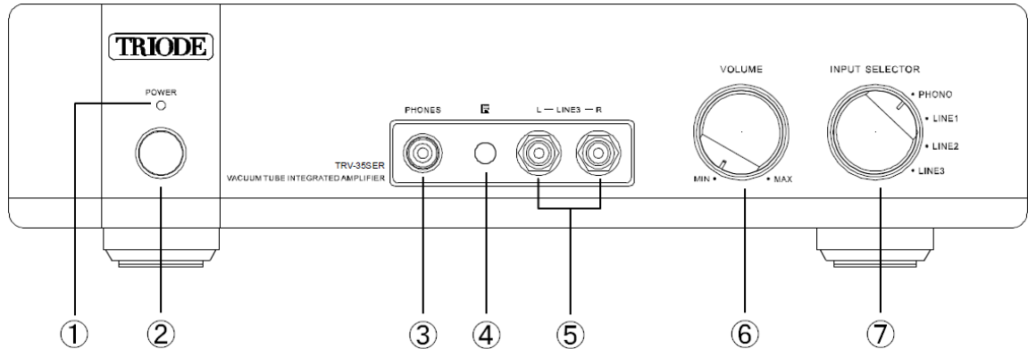
図1 フロントパネル
